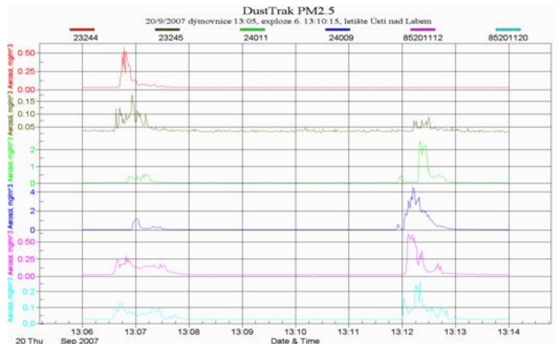
Obrázek 27: Podoba výstupů z laserového fotometru DustTrak – celkový časový průběh koncentrace PM_{2.5} během testu ZÁŘÍ_6 (průchod oblaku aerosolu znázorňují píky vpravo)
