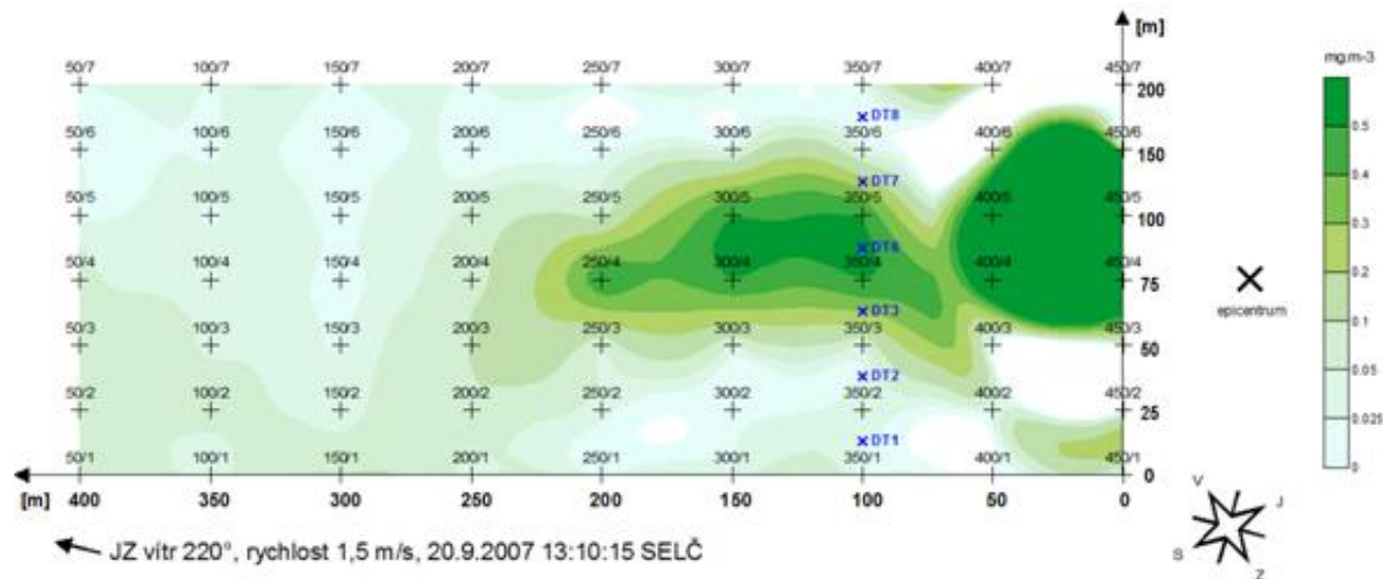
Obrázek 31: Průměrná koncentrace aerosolu během přechodu oblaku v \text{mg}\cdot\text{m}^{-3} pro test ZÁŘÍ_6
